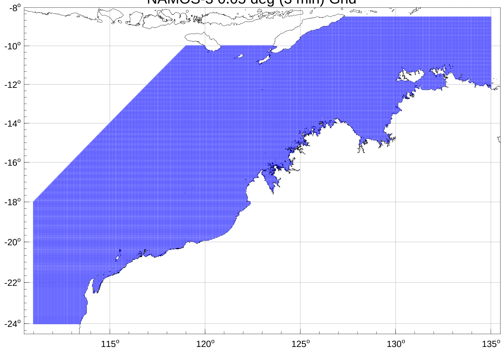
NAMOS-3 0.05 deg (3 min) Grid
